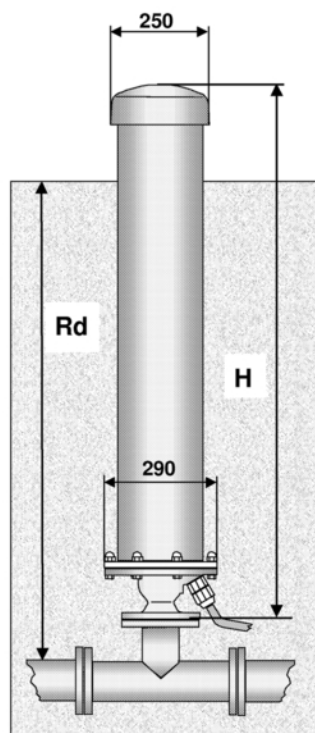
Zabudowa nadziemna
